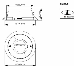
TCGSRR 250 30S/830 C PSU-E WH
